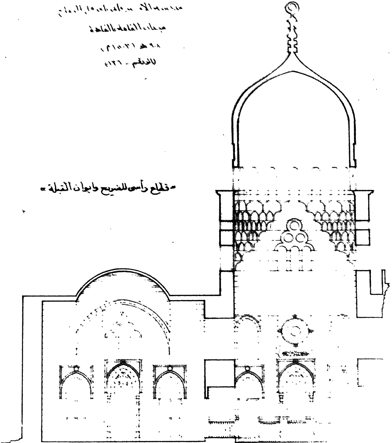
شكل (١٧) يبين قطاع رأسى لضريح واىوان القبلة بمدرسة قانى باى الرماح بميدان القلمة
